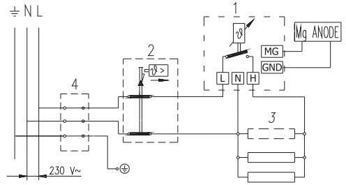
Skema e lidhjes elektrike
